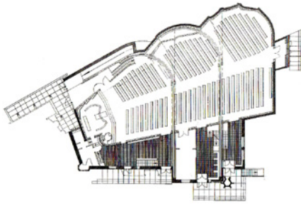
Grundriss Kirche der drei Kreuze Vuoksenniska, Alvar Aalto-Museum
